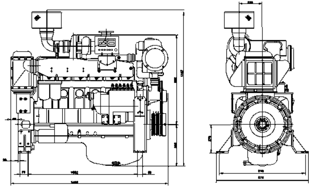
WD618 系列船用柴油機外形尺寸圖
